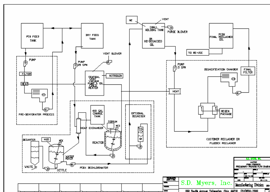
Figura 21: Fluxograma simplificado de processo (SDMYers Inc)
