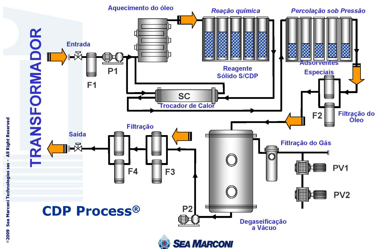
Figura 22: Fluxograma simplificado de processo (SEA Marconi)
