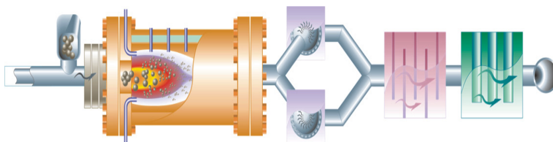
Figura 18: Esquema simplificado do sistema de oxidação à pressão
